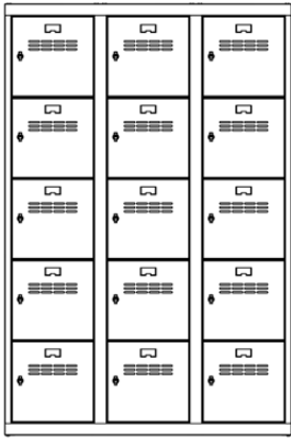
réf. CME543 L.1200 x P.500 x H.1800 mm
