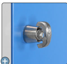
Morillon porte-cadenas débrayable assurant une meilleure résistance à l'effraction par rotation
